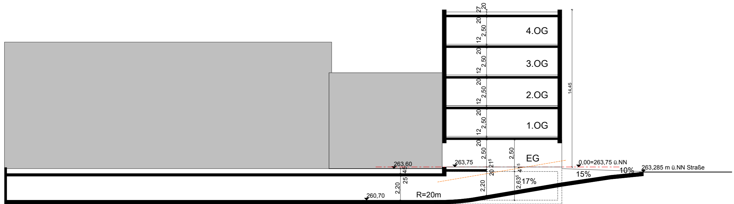
SCHNITT A - LUFTSCHLOSS
